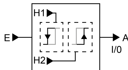
Bild 17: Grenzwertschalter
