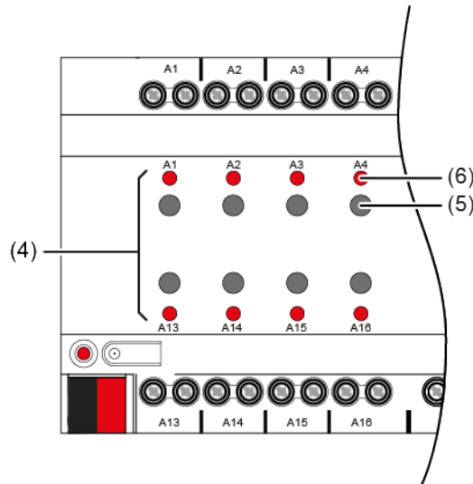
Bild 5: Bedienelemente – Übersicht
