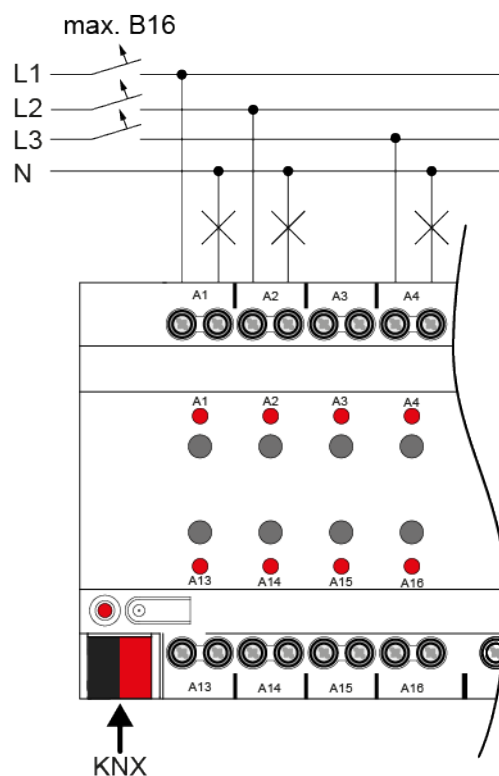
Bild 3: Geräteanschluss (Anschlussbeispiel)
