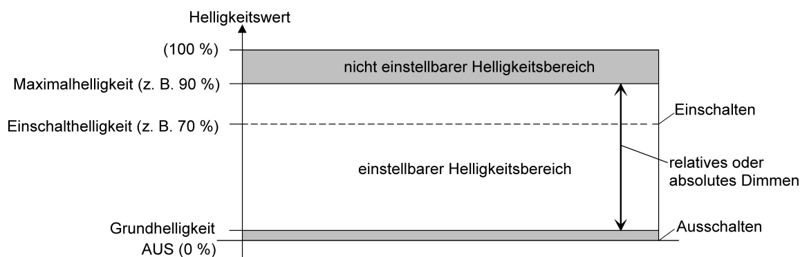
Bild 13: Beispiel eines Helligkeitsbereiches mit Grundhelligkeit
