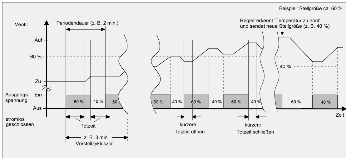
Bild 16: Idealisierter Verlauf des Ventilhubes exemplarisch dargestellt für eine Zykluszeit < Verstellszykluszeit
