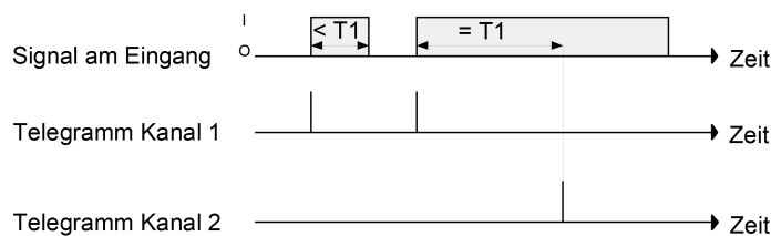
Bild 25: Beispiel zum Bedienkonzept "Kanal 1 und Kanal 2"
